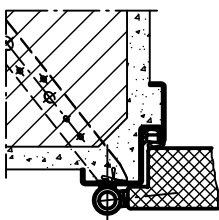
Profil 22 za montažu na zid
