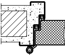
Profil 81
