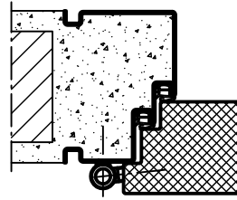
Profil 78
