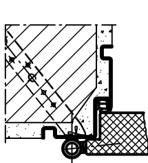
Profil 50 za montažu na zid
