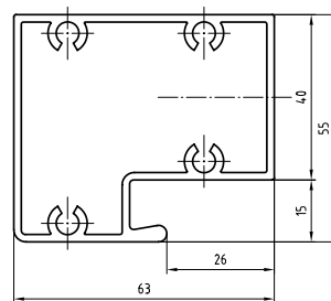
Alumijski potporanj profil 904 profil za priključak na strop ili pod
