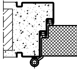
Profil 77
