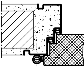
Profil 38
