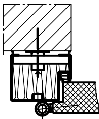
Prednji dovratnik za montažu klinovima
