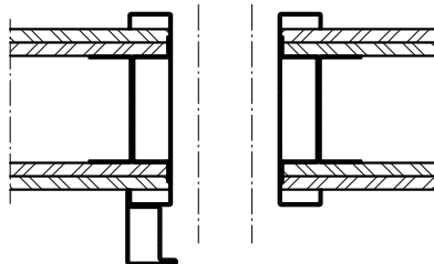
Dovratnik za klizna vrata, koja idu ispred zida
