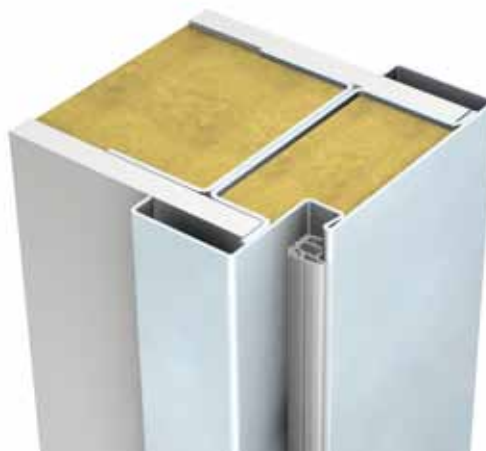
Slika: profil 42 za montažu na zid sa profilom
