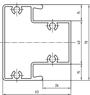
Alumijski potporanj profil 992
