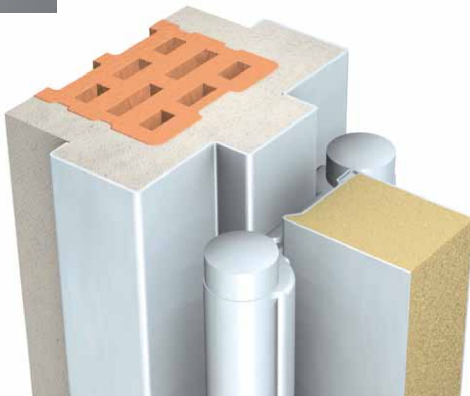
Slika: Profil 506 za montažu na zid
