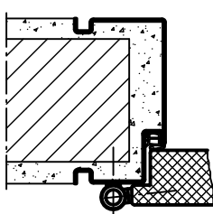
Profil 46 za montažu na zid
