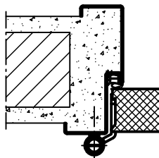
Profil 41
