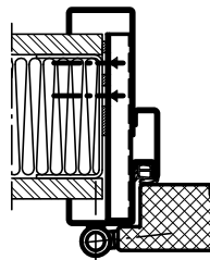
Profil 102
