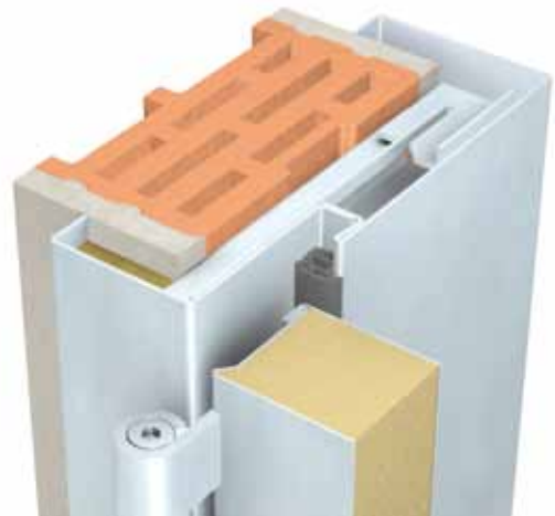
Slika: profil 101 za montažu na zid
