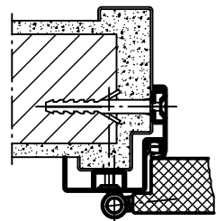
Profil 70
