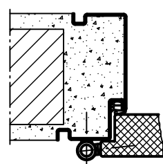
Profil 48 za montažu na zid
