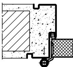
Profil 47
