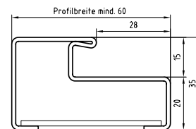
Alumijski potporanj profil 994 profil za pod za ostakljenje sa strane
