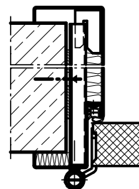
Profil 106
