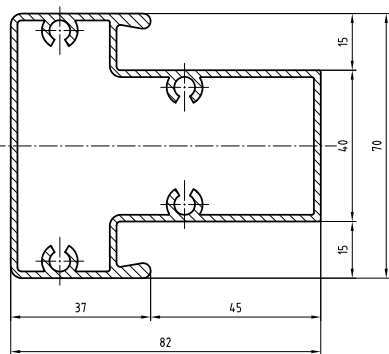
Alumijski potporanj profil 991
