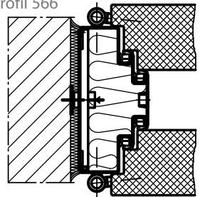
Profil 566
