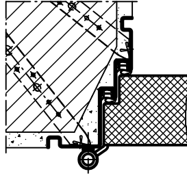
Profil 39
