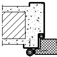
Profil 24 za montažu na zid
