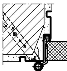
Profil 49
