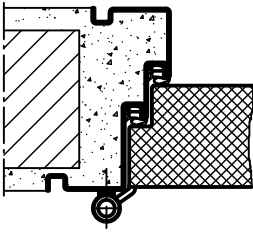
Profil 37
