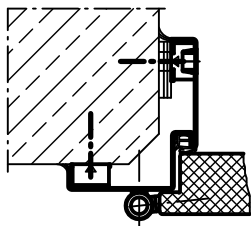
Profil 24 a montažu klinovima
