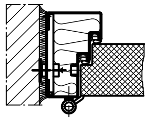
Profil 79
