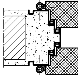
Profil 565
