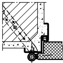
Uglasti dovratnik za montažu klinovima, a i za montažu na zid
