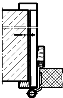
Profil 107
