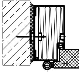
Profil 56 za montažu klinovima
