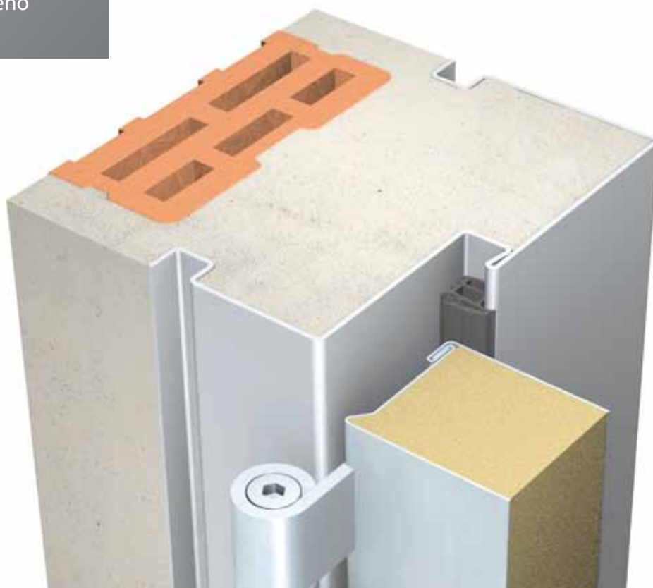
Slika: Profil 45 za ugradnju na zid
