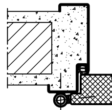
Dovratnik koji obuhvaća, za montažu na zid, a i za standardni zid
