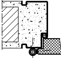
Profil 46
