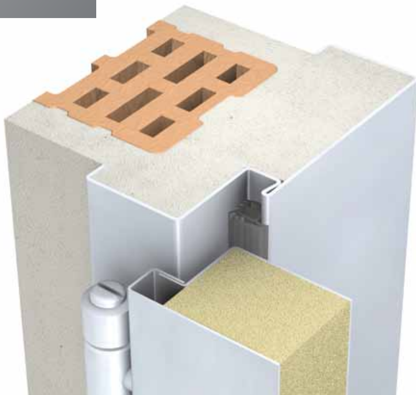
Slika: Profil 42 za montažu na zid
