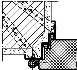
Profil 84
