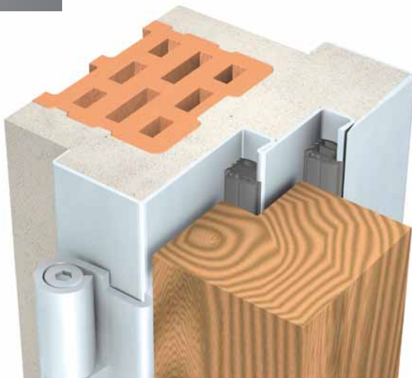
Slika: Profil 81, za montažu na zid
