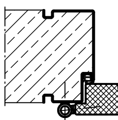
Profil 46 za gradnju s oplatom
