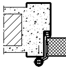
Profil 43
