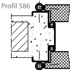
Profil 586
