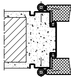
Profil 564
