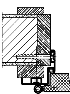
Profil 72 za montažu na zid
