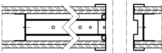
Dovratnik za klizna vrata, koja ulaze u zid
