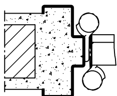
Profil 506
