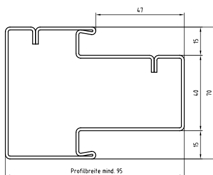
Čelični potporanj profil 901 (min. širina 95)
