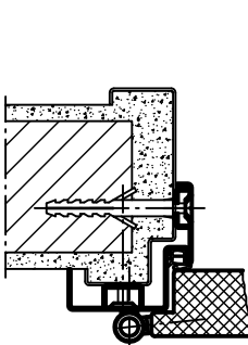
Profil 70 za montažu vijcima
