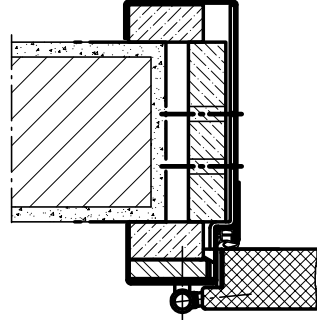
Profil 66 za montažu vijcima
