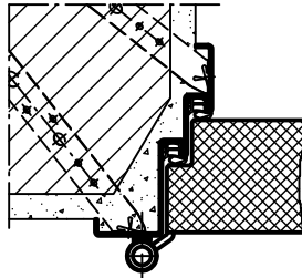
Profil 83
