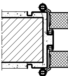
Profil 563
