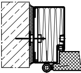
Profil 56
