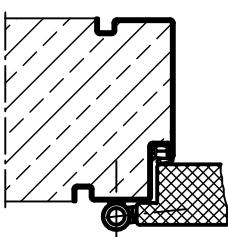
Profil 48 za gradnju s oplatom
