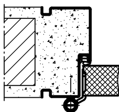
Profil 45
