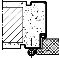
Profil 48 *
