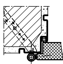
Profil 50
