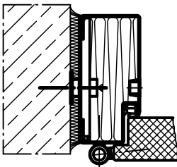
Profil 44 za montažu klinovima
