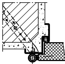
Uglasti dovratnik za montažu na zid
