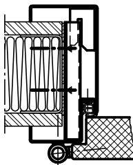
Profil 101
