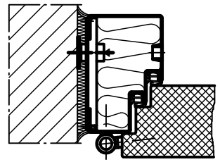
Profil 80
