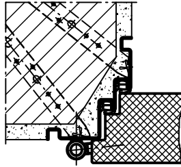
Profil 40
