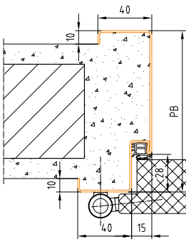
Profil 42_M - str. 10, 14 BRMB = DLB + 100 mm BRMH = DLH + 50 mm
