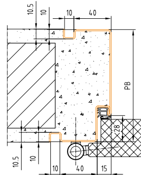
Profil 48_M - str. 12, 14 BRMB = DLB + 120 mm BRMH = DLH + 60 mm
