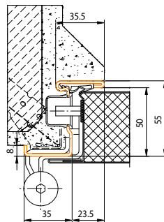
Profil 375_M - str. 26 BRMB = DLB + 90 mm BRMH = DLH + 45 mm (90 mm bei OEL1, OEL2)
