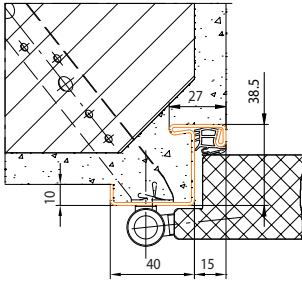
Profil 20_M - str. 17 BRMB = DLB + 70 mm BRMH = DLH + 35 mm
