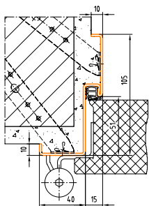
Profil 90_M - str. 29 BRMB = DLB + 50 mm BRMH = DLH + 25 mm
