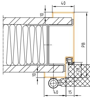
Profil 42_G - str. 11, 14 BRMB = DLB + 96 mm BRMH = DLH + 48 mm
